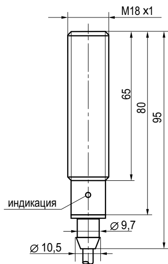
Габаритный чертеж.
